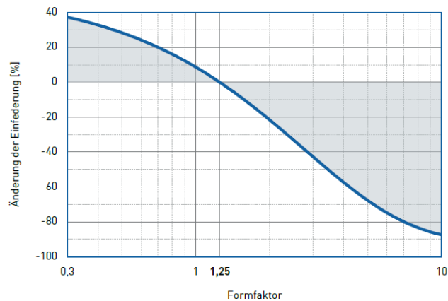
Einfederung
