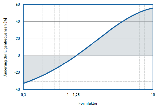
Eigenfrequenz
